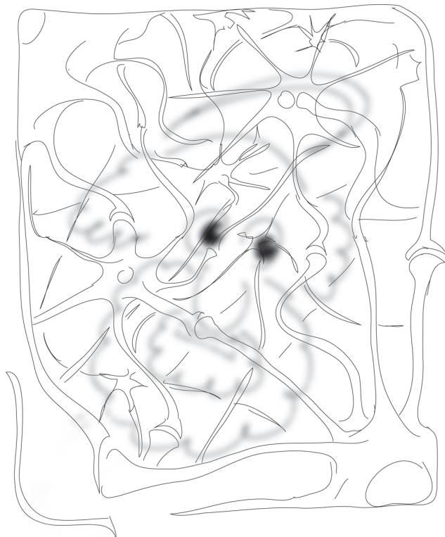
Нейронная сеть.
